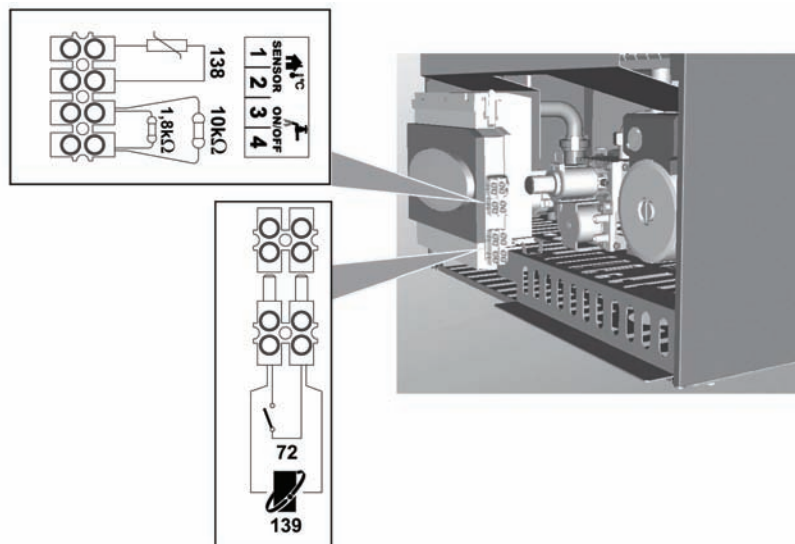
fig. 18 - Accesul la panoul de borne
