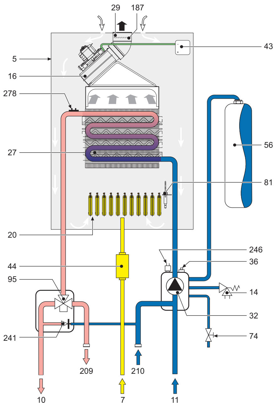
fig. 32 - Circuitul hidraulic
