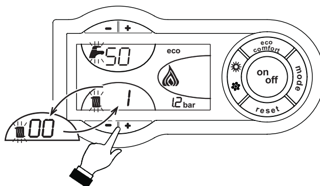
fig. 26 - Modul TEST (putere de încălzire = 100%)
