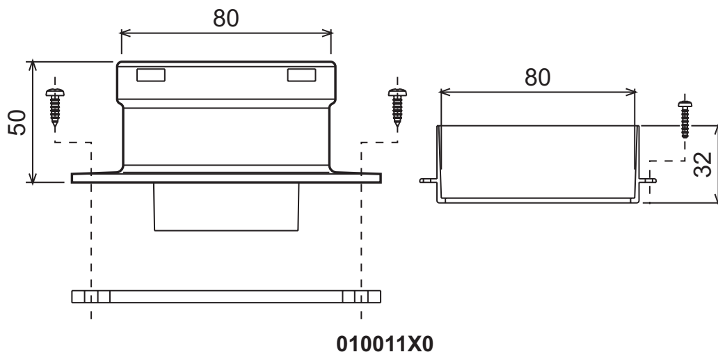
fig. 24 - Accesoriu de plecare pentru conducte separate
