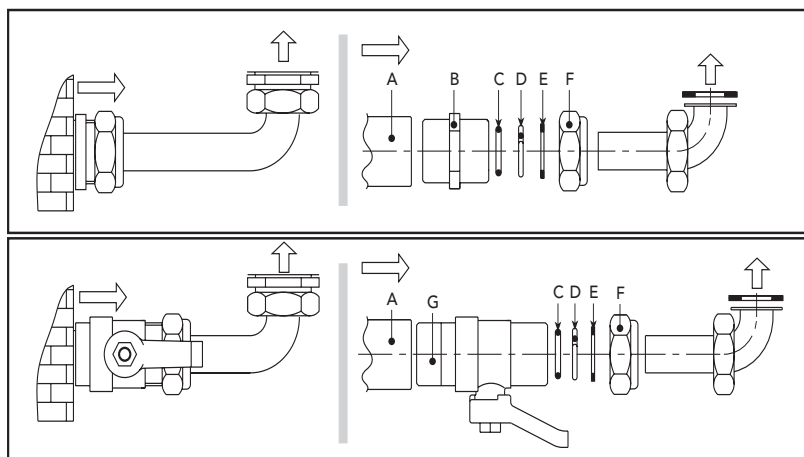
fig. 17 - Kit de racordare
