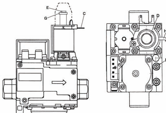
fig. 27 - Valvă de gaz
