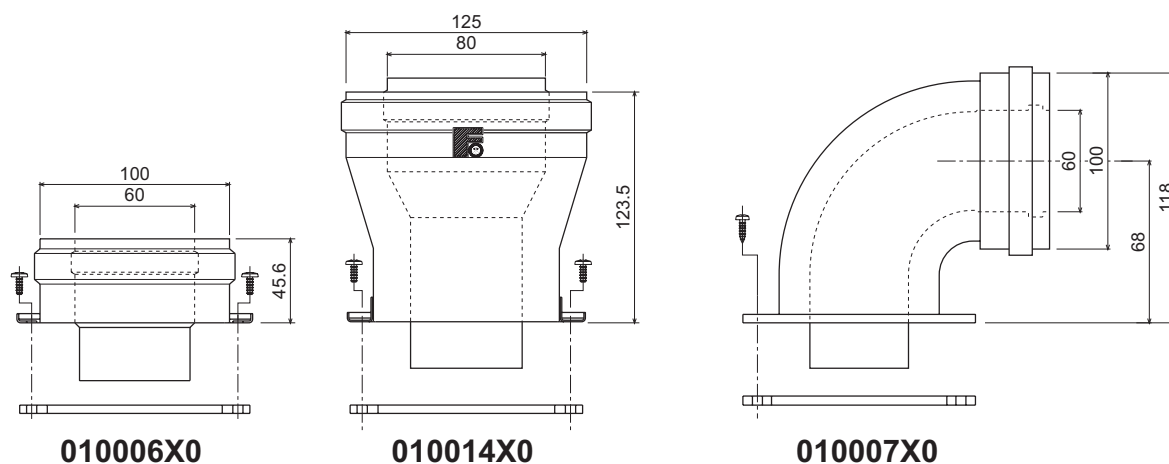
fig. 22 - Accesorii de plecare pentru conducte coaxiale
