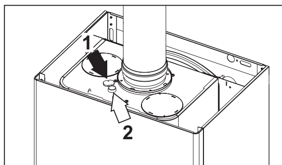
fig. 29 - Analizarea gazelor arse
