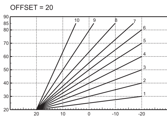
fig. 14 - Exemplu de deplasare paralelă a curbelor de compensare
