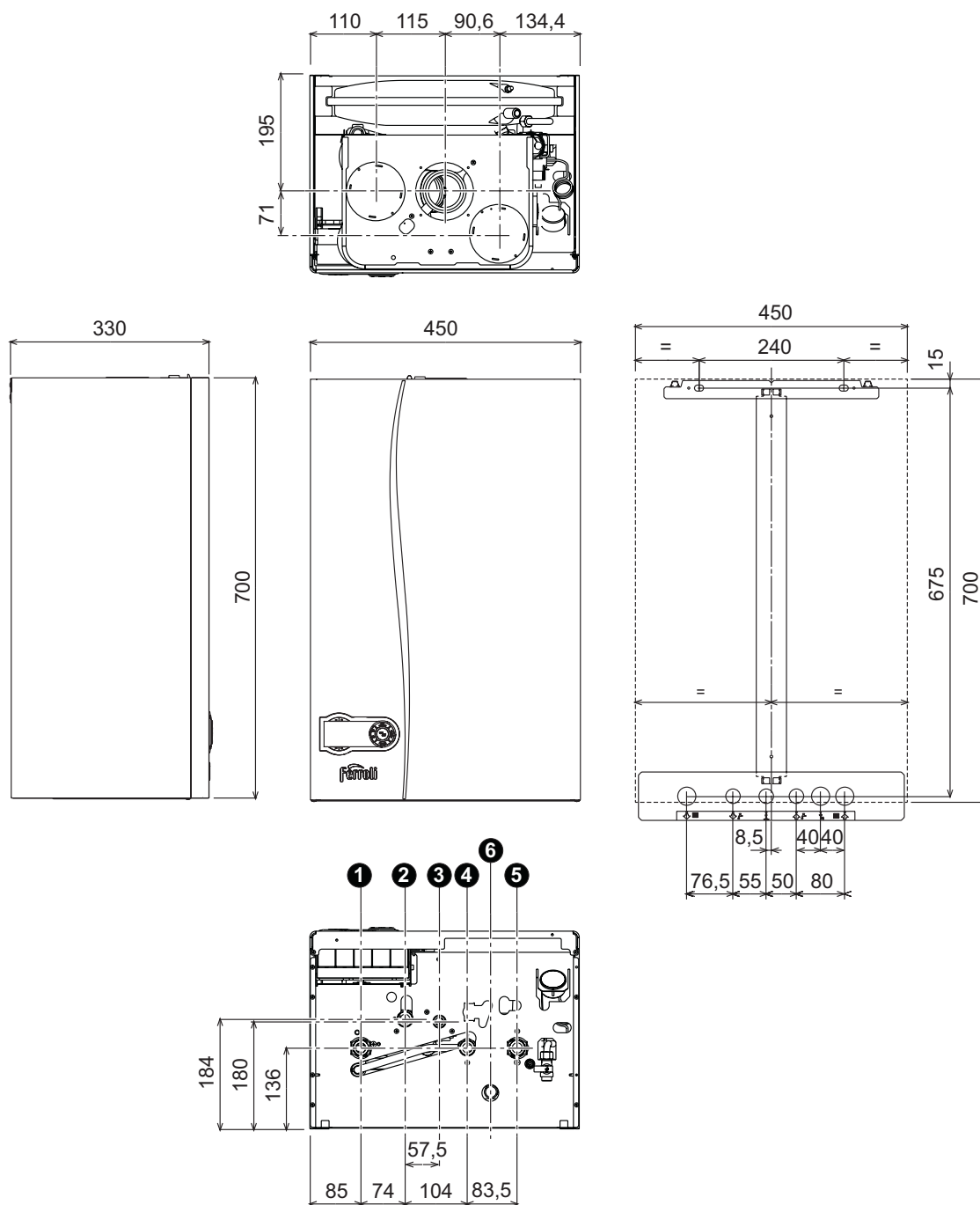
fig. 30 - Dimensiuni și racorduri
