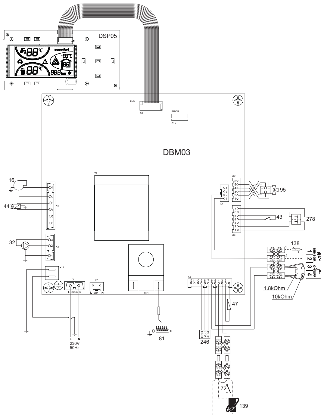
fig. 33 - Schemă electrică
