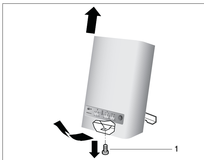
Fig. 15 Se scoate capacul
