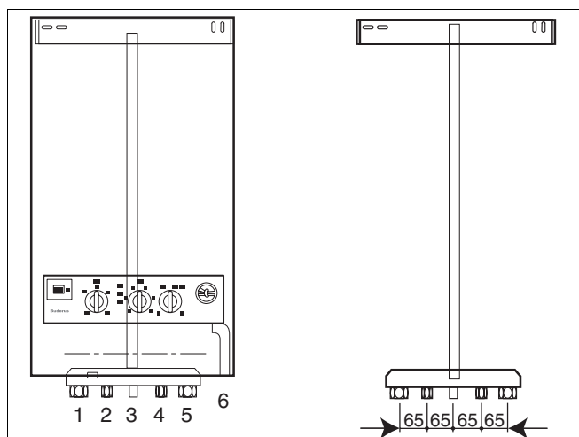
Fig. 16 Montaj
