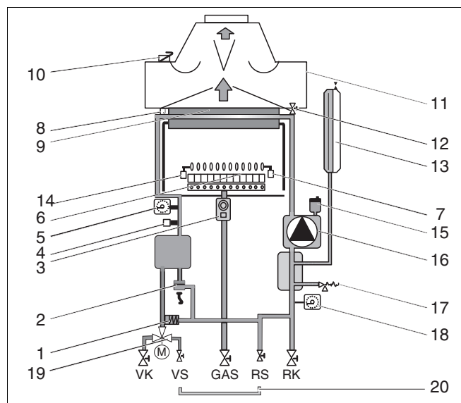
Fig. 4 Schema de funcționare Logamax U004 cu robinet cu 3 căi
