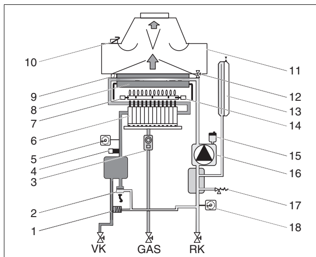
Fig. 2 Schema de funcționare Logamax U104
