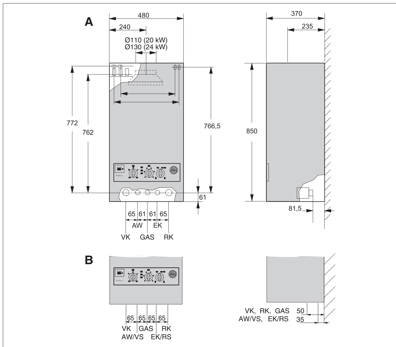
Fig. 8 Dimensiunile cazanului de perete
