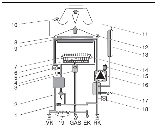
Fig. 3 Schema de funcționare Logamax U004 cu limitator debit apă
