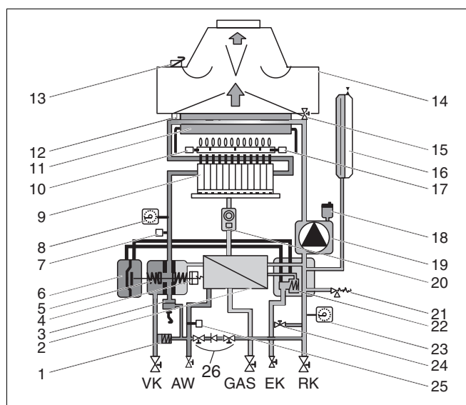
Fig. 7 Schema de funcționare Logamax U104K cu limitator debit apă (FR) sau instalație de umplere (IT/TR)
