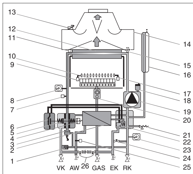
Fig. 6 Schema de funcționare Logamax U004K cu limitator debit apă (FR) sau instalație de umplere (IT/TR)
