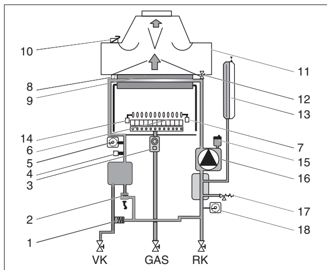
Fig. 1 Schema de funcționare Logamax U004
