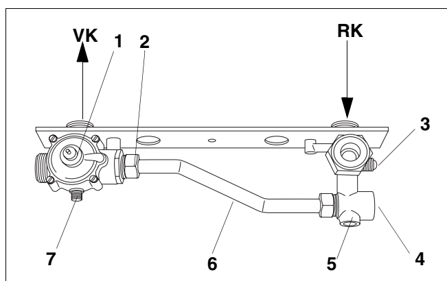
Fig. 26 Unitatea hidraulică la aparatul simplu
