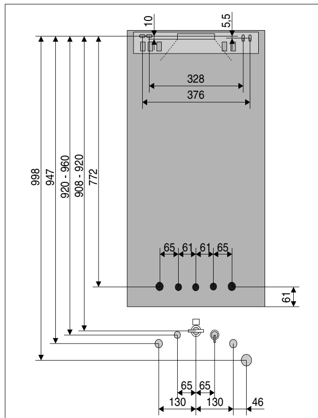
Fig. 11 Compatibilitate cu Junkers ZWR (aparat combi)
