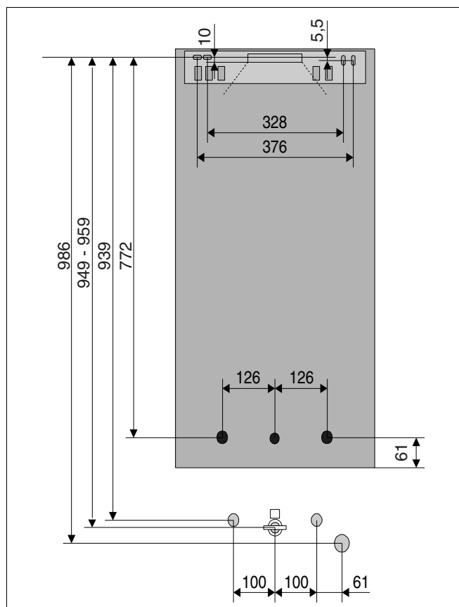
Fig. 10 Compatibilitate cu Vaillant VC (aparat simplu)
