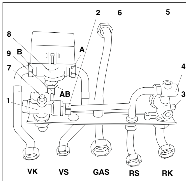
Fig. 27 Unitatea hidraulică la aparatul simplu cu robinet cu 3 căi
