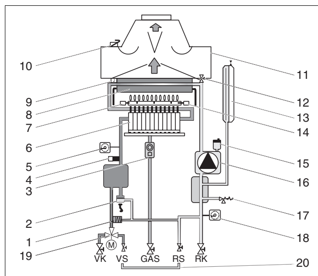
Fig. 5 Schema de funcționare Logamax U104 cu robinet cu 3 căi
